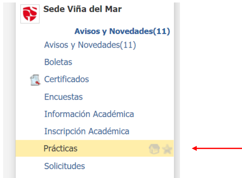
Figura N° 1: Menú IEBVirtual
